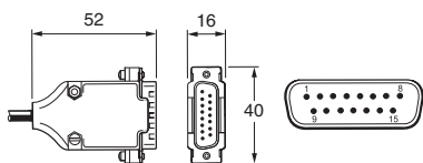
15 針 D 型插頭 (端子代碼 D)
