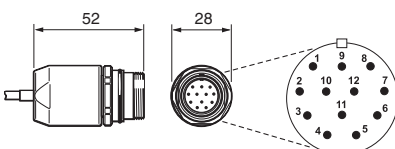
12 針圓形耦合接頭 (端子代碼 W)
