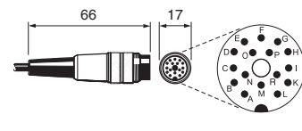
16 針串聯連接器插頭 (端子代碼 X)
