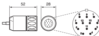
12 針圓形插頭 (端子代碼 R)
